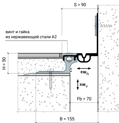
MANGRA 6250-070/AL, h = 50 мм, Угол
