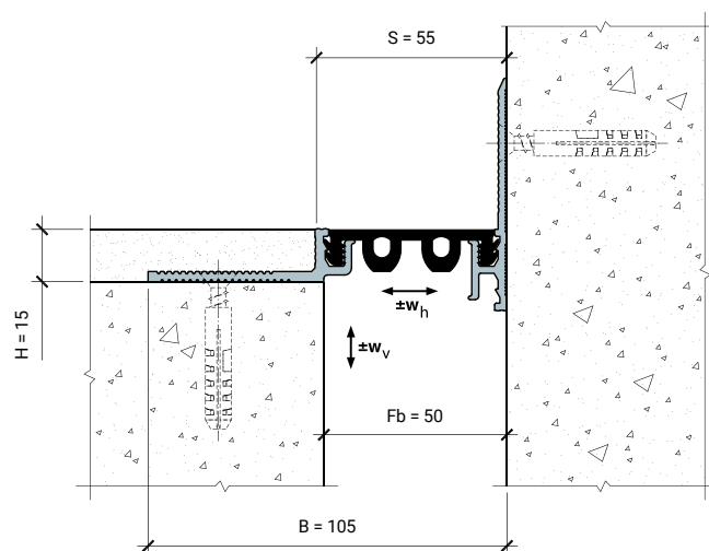
MANGRA 3320-050, h = 15 мм, Угол, вставка гладкая
