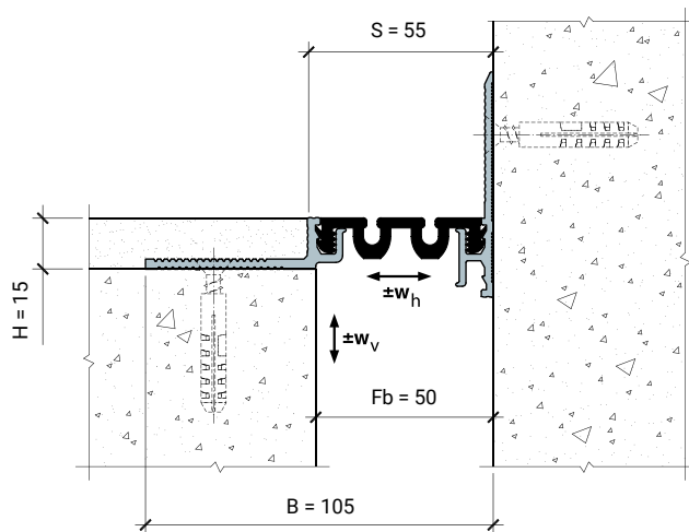
MANGRA 3320 - 050 , h = 15 мм , Угол
