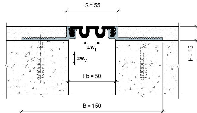
MANGRA 3320-050, h = 15 мм
