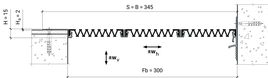
MANGRA 3210-300 Угол
