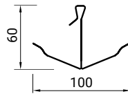
L-клипса для швов шириной 35–50 мм
