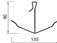
XL-клипса для швов шириной 50–100 мм
