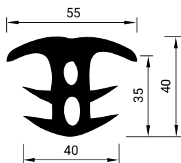
MANGRA 2420-030 для шва 23–34 мм
