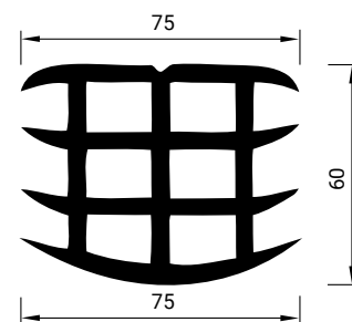
MANGRA 2420-060 для шва 50–65 мм
