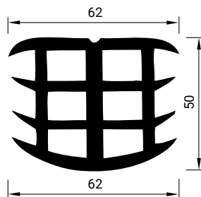
MANGRA 2420-050 для шва 43–52 мм
