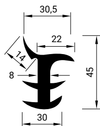
MANGRA 2420-020, Угол для шва 15–25 мм
