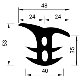
MANGRA 2420-030, Угол для шва 23–34 мм
