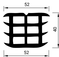
MANGRA 2420-040 для шва 37–43 мм
