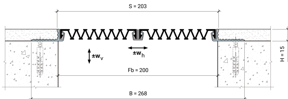
MANGRA 3220-200
