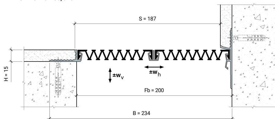
MANGRA 3220-200, Угол
